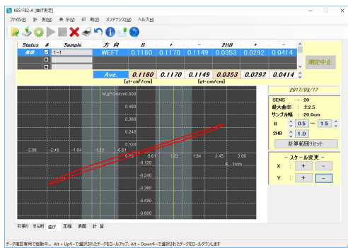
▲曲げ特性
